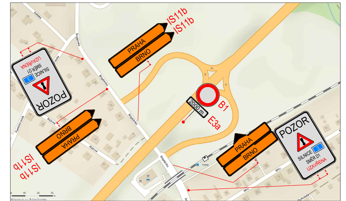
dopravní značení v prostoru MÚK Čerčany
